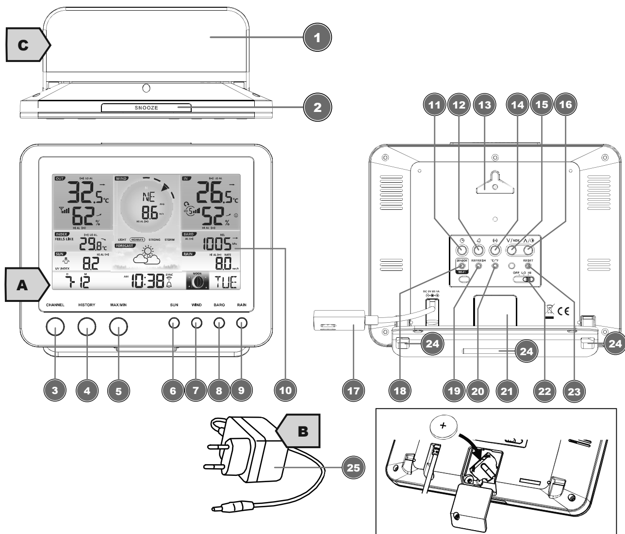
Fig. 1: Tutti i componenti della centralina
