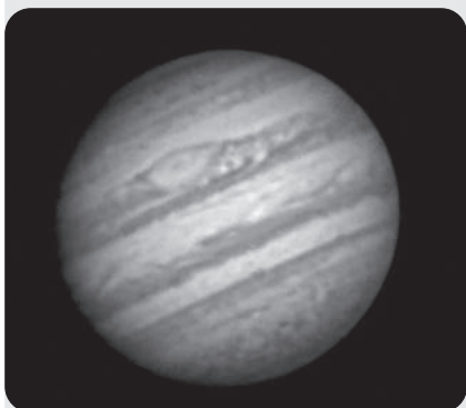
Fig. 43a: El planeta Júpiter, mostrado aquí con gran aumento. Las estructuras de nubes se pueden ver claramente. Las cuatro grandes lunas pueden observarse en una posición diferente cada noche.
